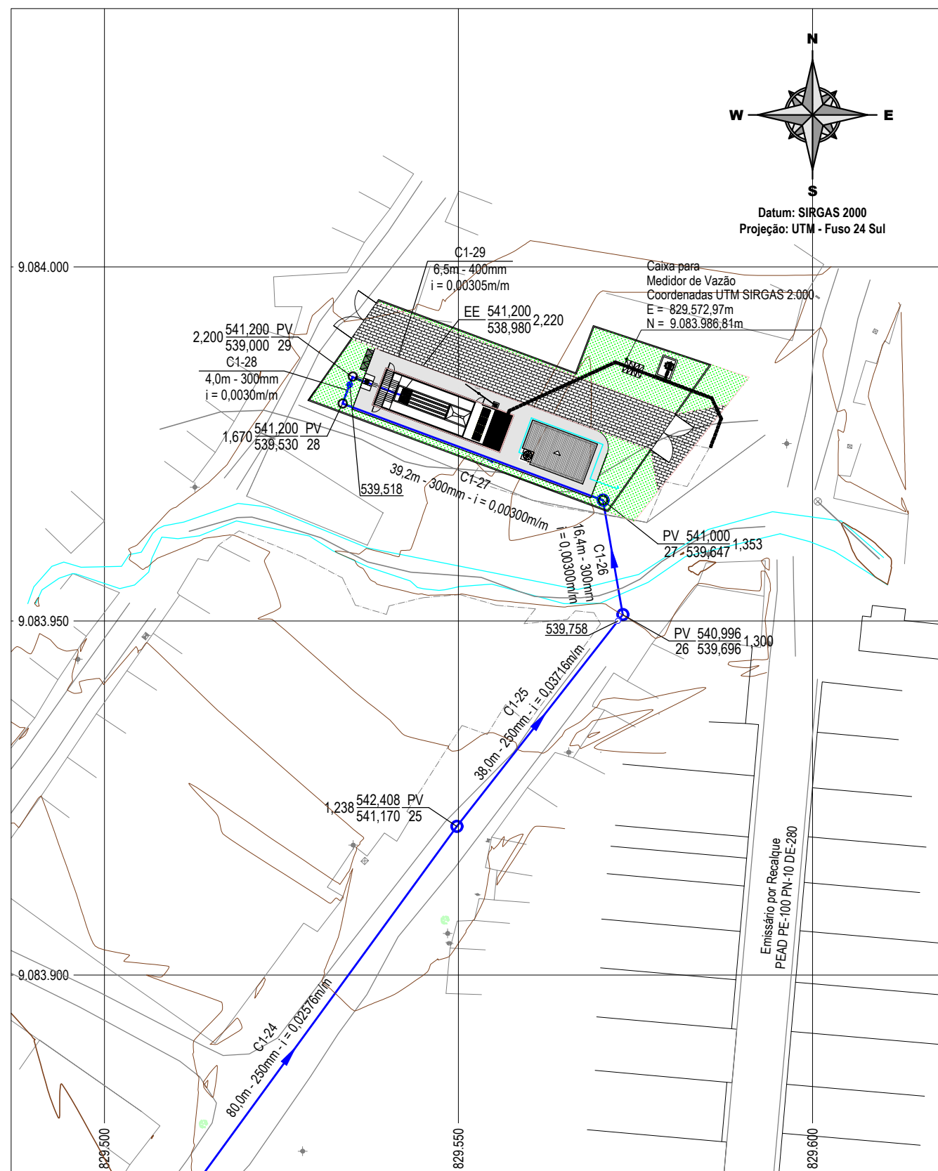
Planta de Situação Escala 1 : 750
