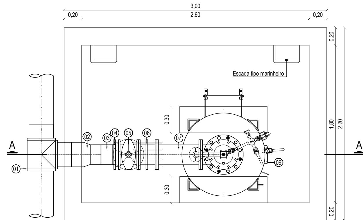
Tanque Hidropneumático - Planta Baixa Escala 1 : 25
