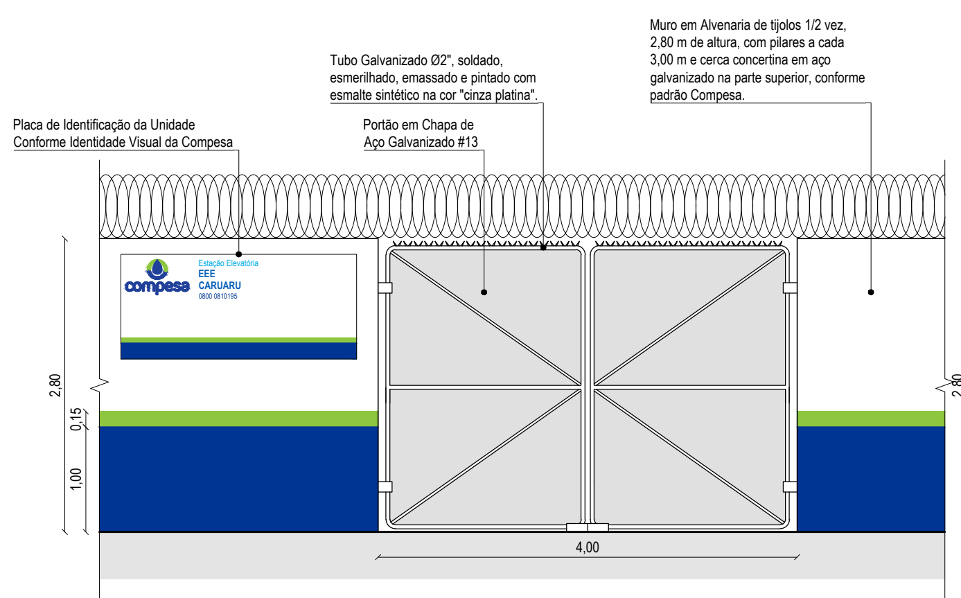
Fachada Principal Escala 1 : 50
