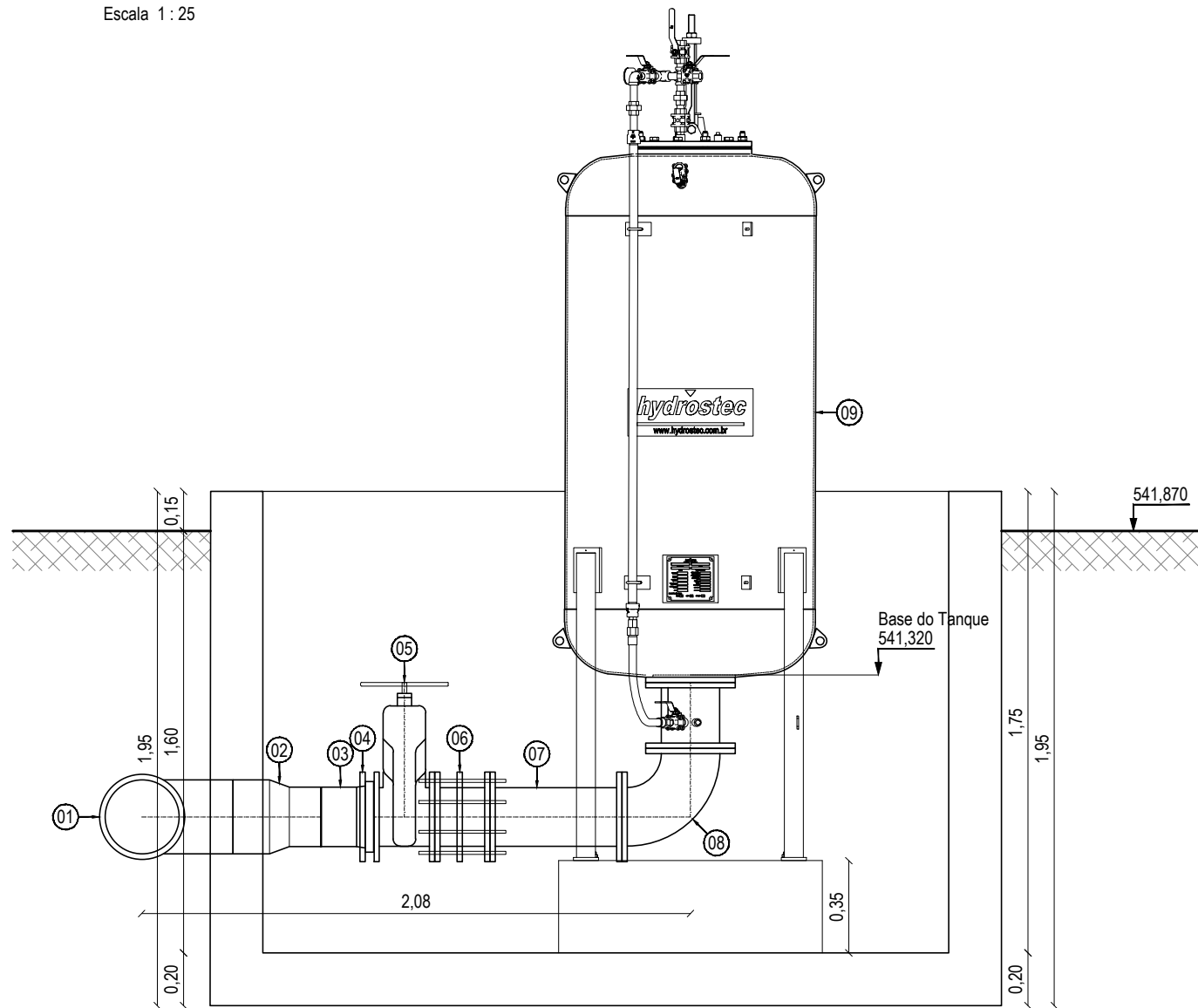
Tanque Hidropneumático - Corte A - A Escala 1 : 25
