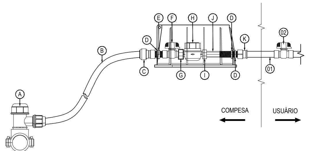
Detalhe Ligação Predial Sem Escala
